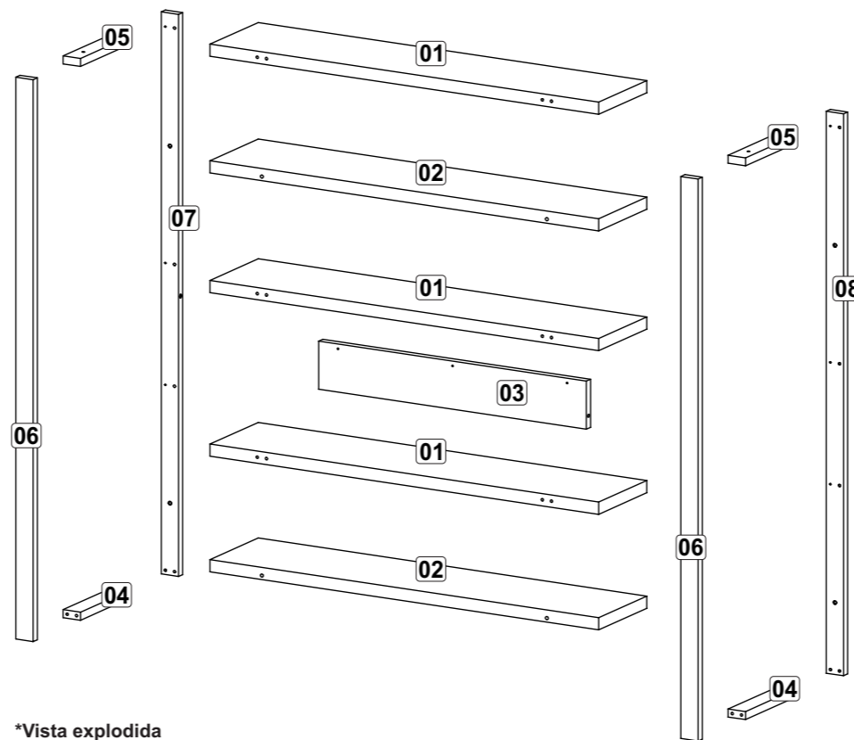
*Vista explodida
